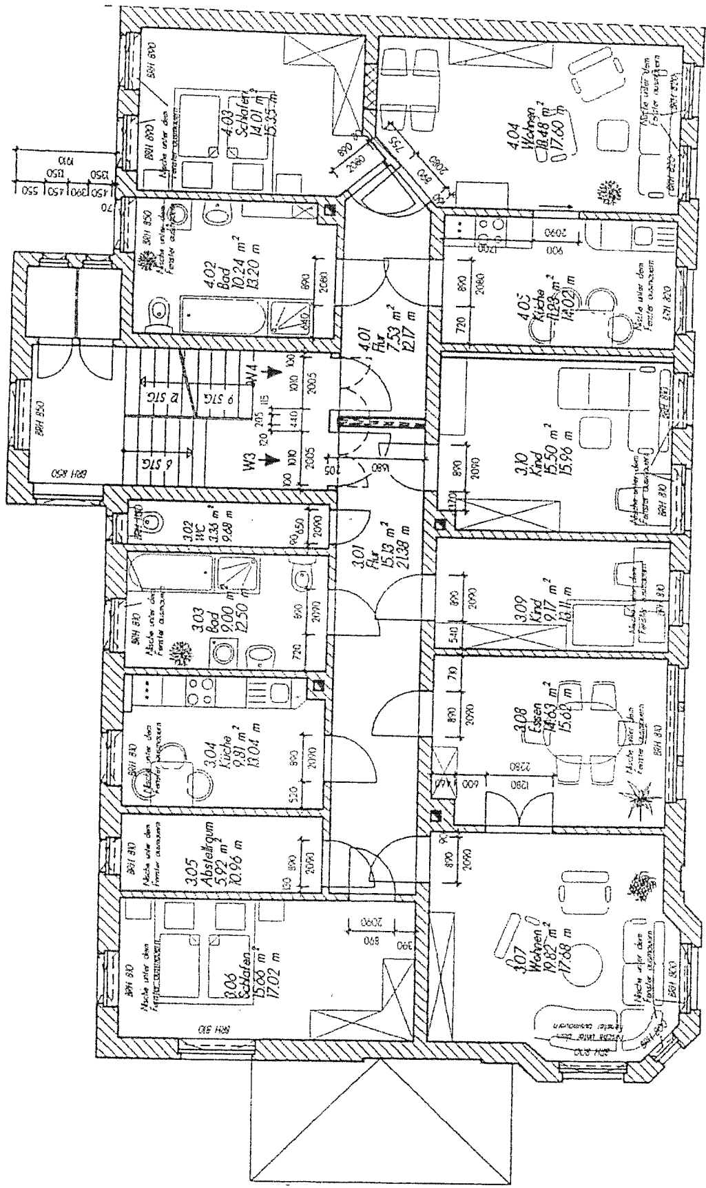
1. Obergeschoss
